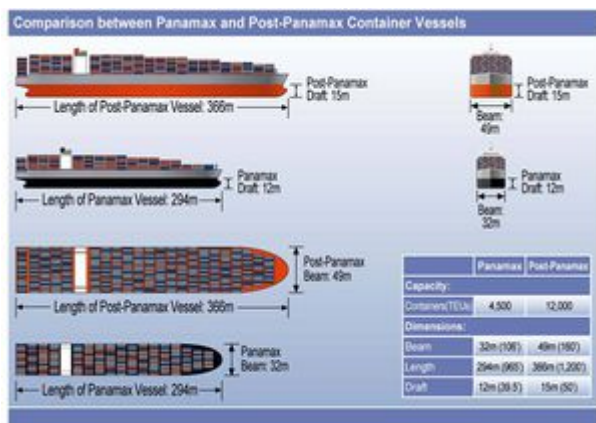
Comparación buques Portacontenedores Panamax y Post-Panamax. Autoridad del Canal de Panama, 2006.
